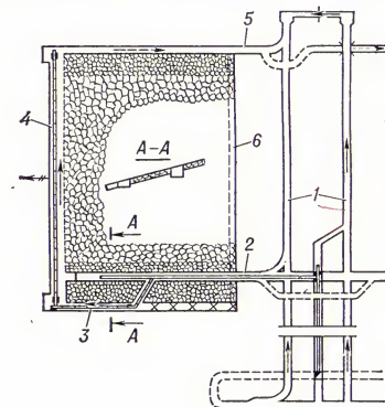
Рис. 10. Сплошная система разработки «лава — этаж»: 1 — наклонные выработки; 2 — этажный конвейерный штрек; 3 — просек; 4 — очистной забой (лава); 5 — этажный вентиляционный штрек; 6 — разрезная печь.
